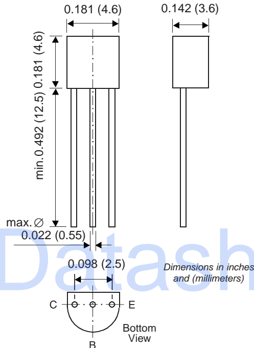
TO-226AA (TO-92)
