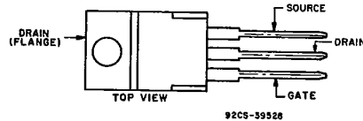
JEDEC TO-220AB
